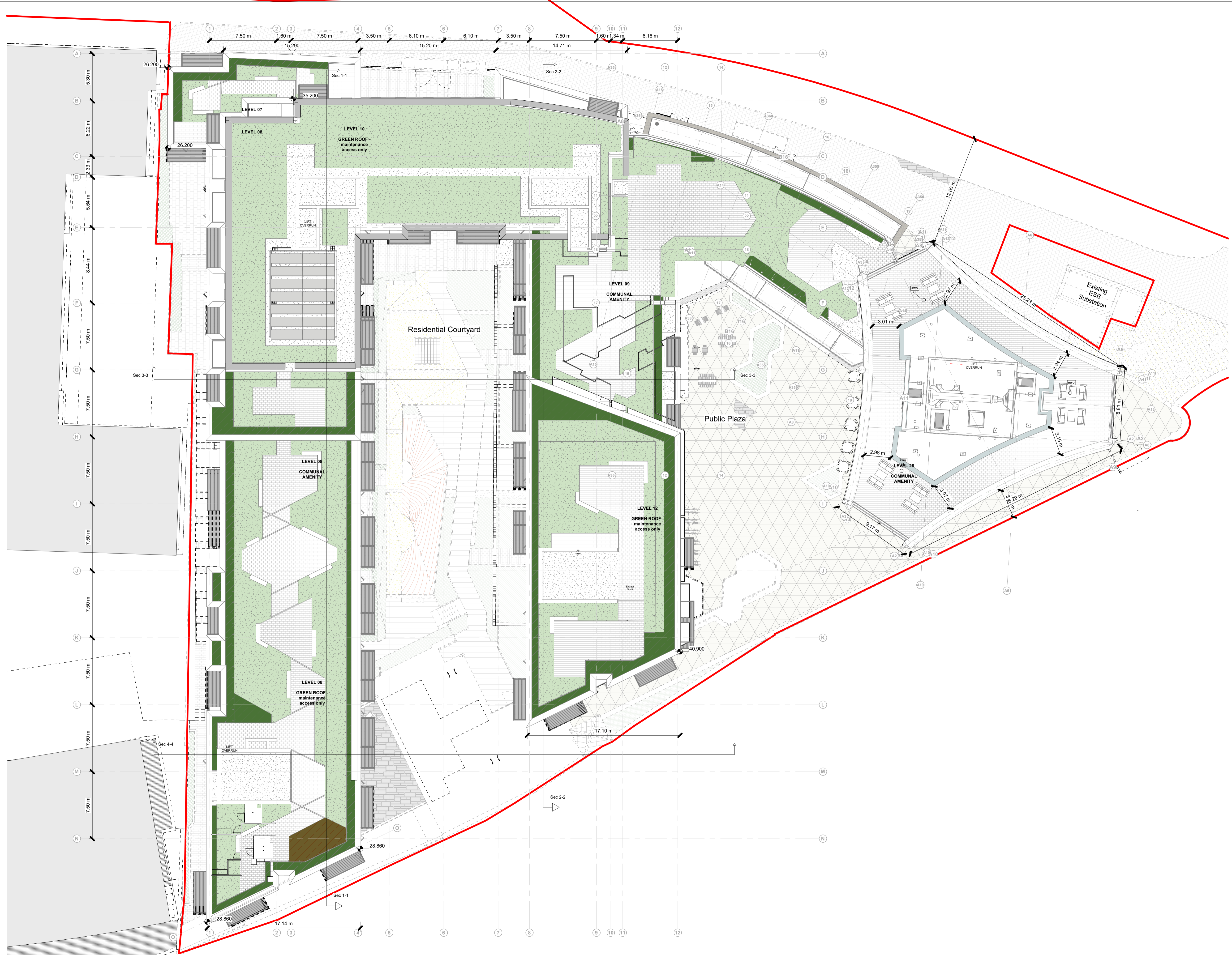
RF - Roof Plan 1 : 200
