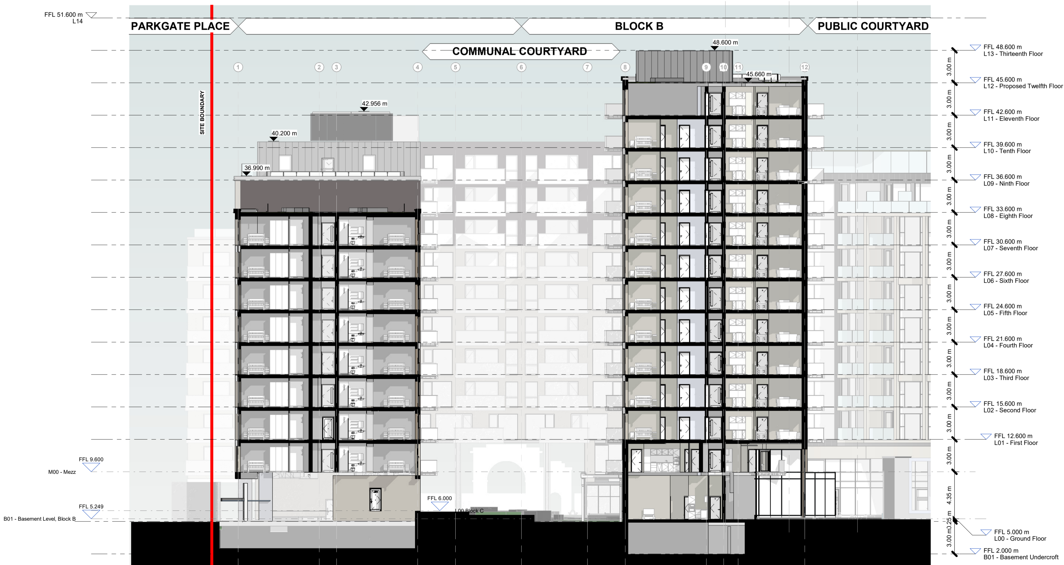
Section C_4-4 1 : 200
