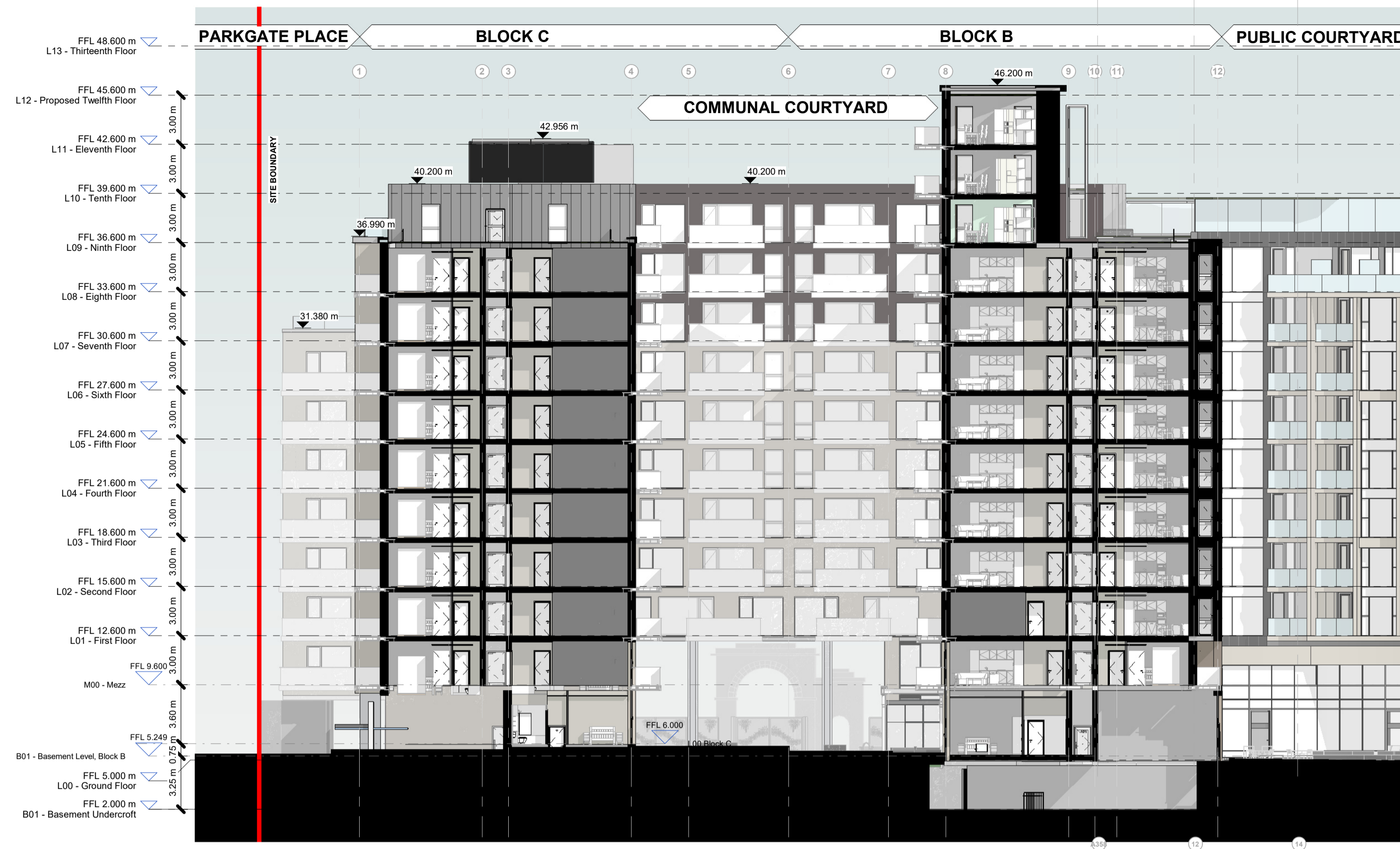
Section BC 3-3 1 : 200
